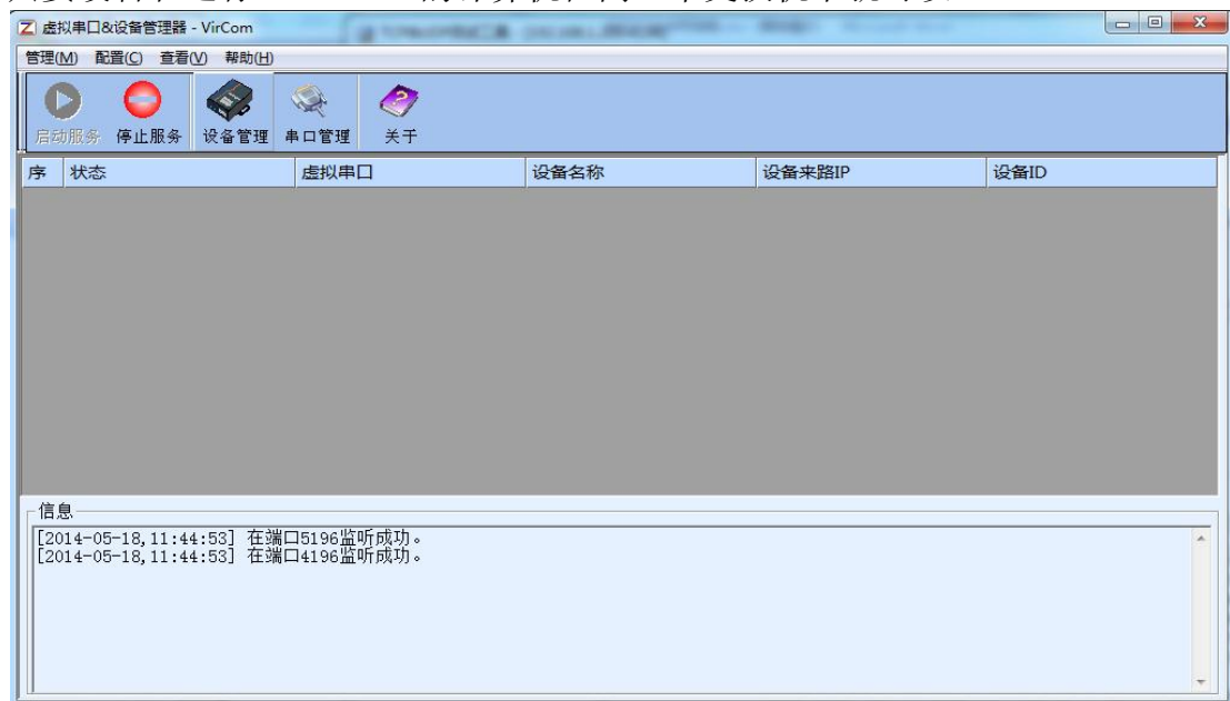
图 14 ZLVircom 主界面
