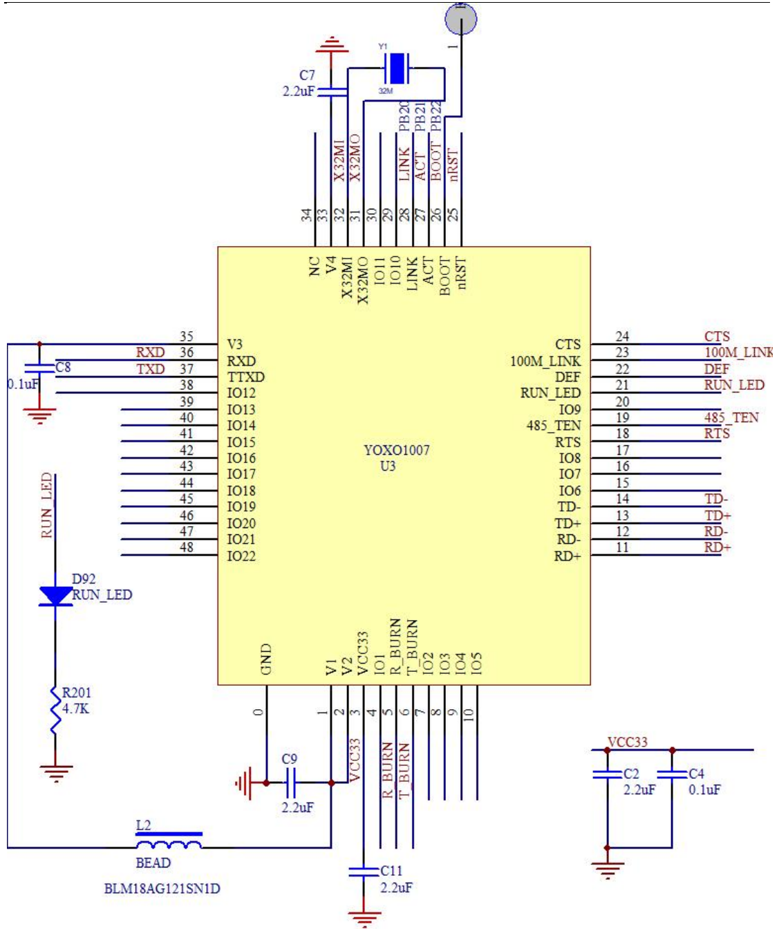
图 9 YOXO1007 原理图核心部分
