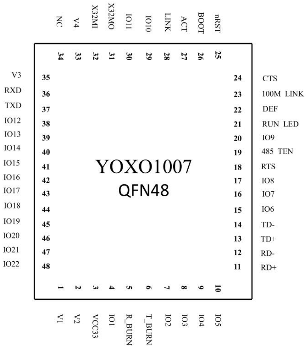
图 7 YOXO1007 引脚图
