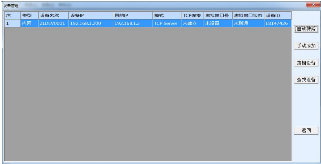
图 15 设备列表
