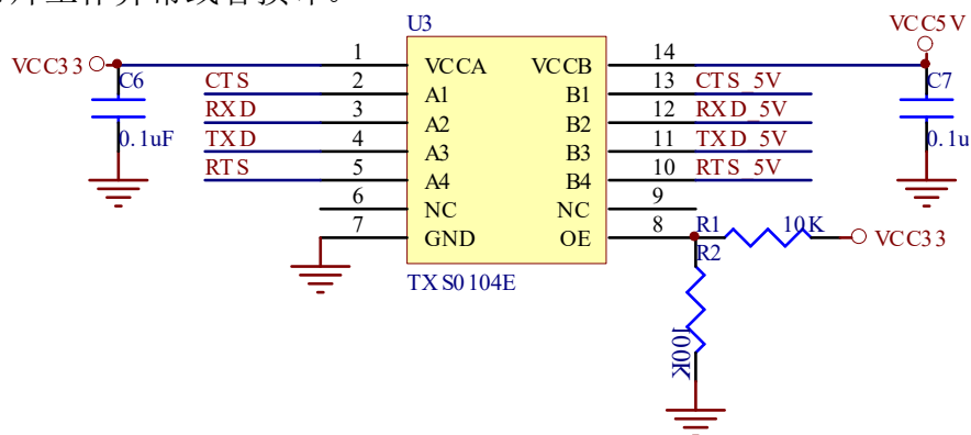
图 13 YOXO1007 原理图 IO 接口电平转化部分
