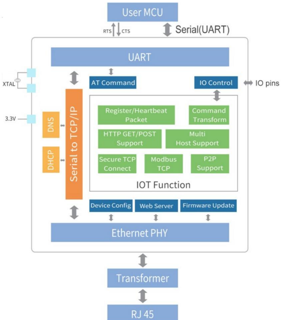
图 2 YOXO1007 方框图
