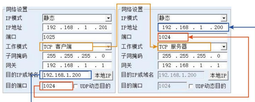
图 26 TCP 设备对联参数配置
