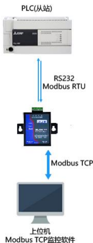
图 34 存储型 Modbus 网关工作方式
