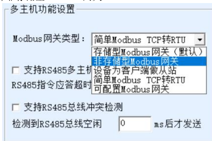
图 27 禁用存储型功能
