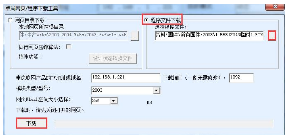
图 42 ZLSN2003 固件升级方法
