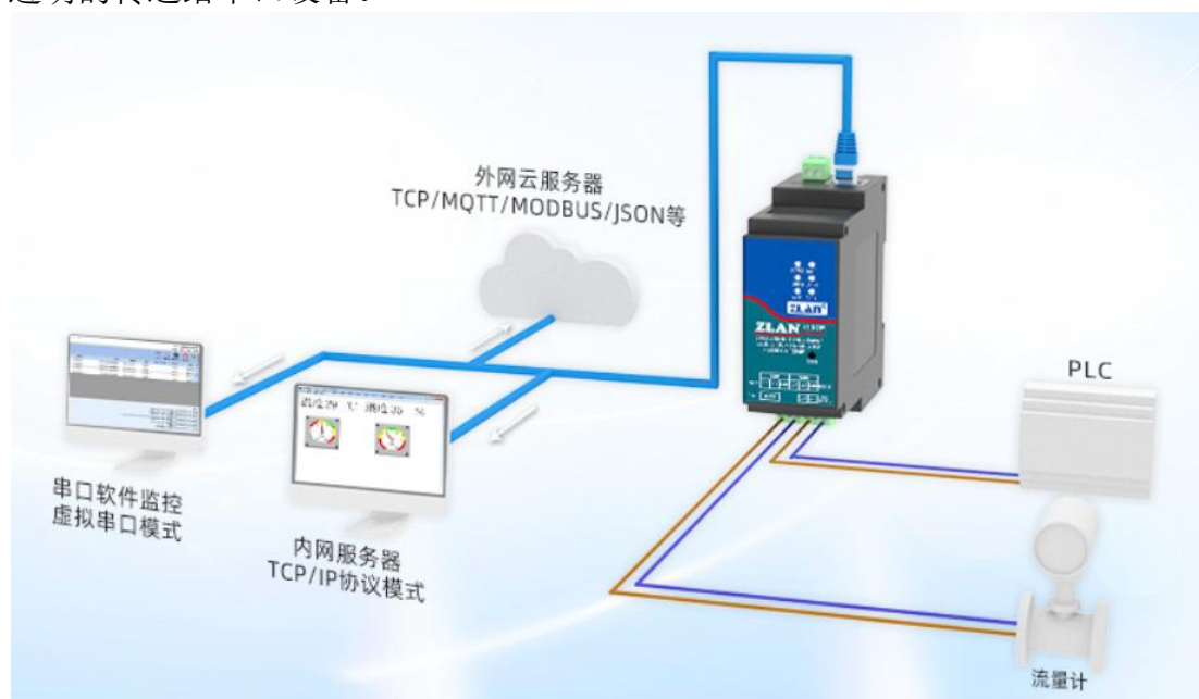
图 2 连接示意图
