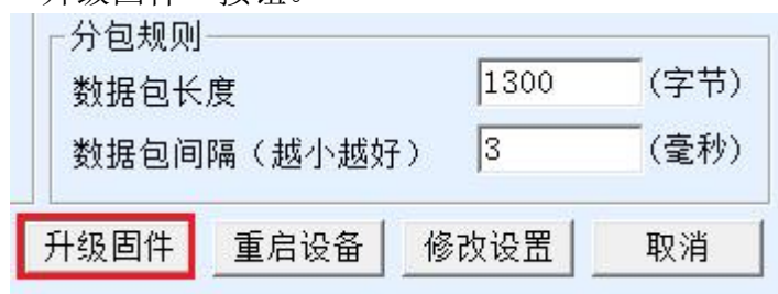
图 41 升级按钮
