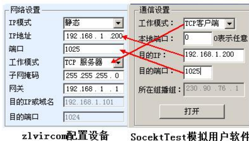
图 21 串口服务器作为服务端
