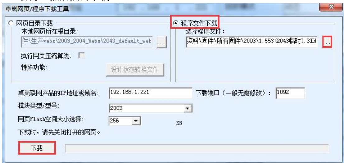
图 47 ZLSN2007 固件升级方法
