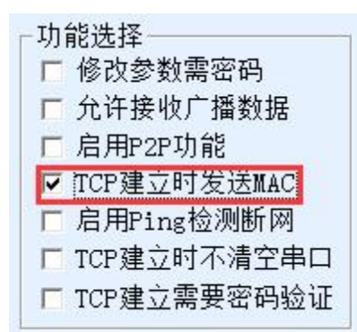
图 36 连接上发送 MAC 地址
