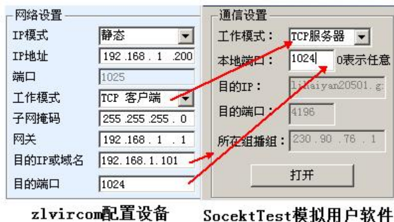
图 18 串口服务器作为客户端
