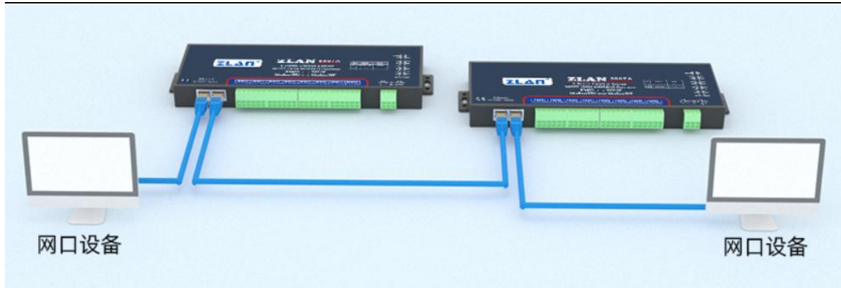
图 50 ZLAN5807A 级联方法
