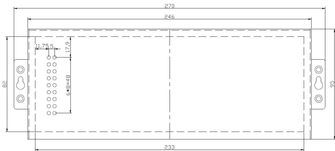
图 52 ZLAN5807A 安装尺寸
