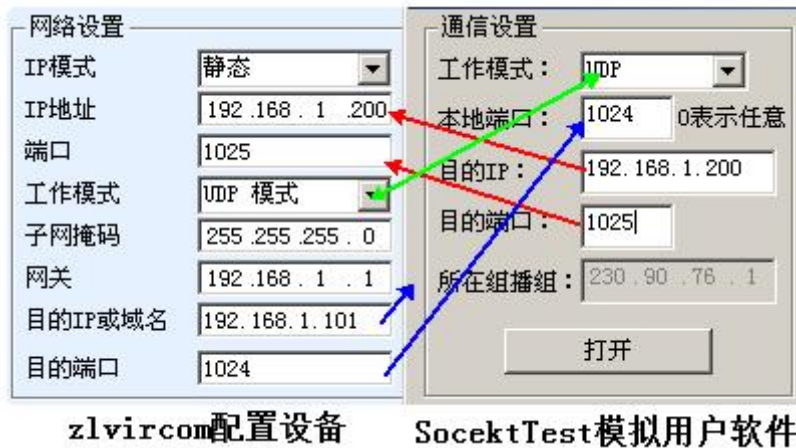
图 23 UDP 模式参数配置
